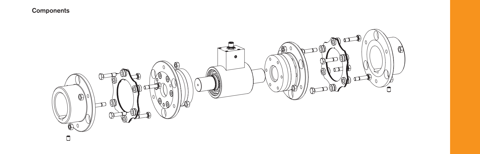
DATAFLEX® 32
