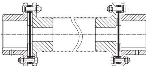
Type NNW (see page 172)
