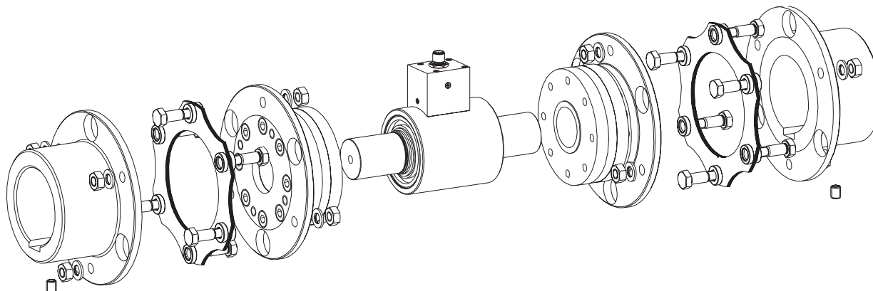
DATAFLEX® 42
