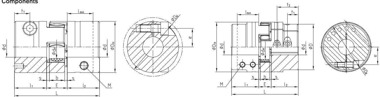
ROTEX® 19 - 28
