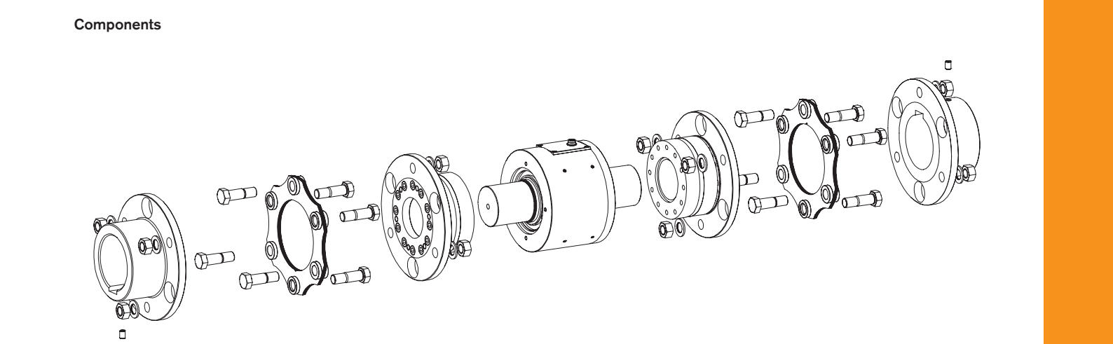
DATAFLEX® 85
